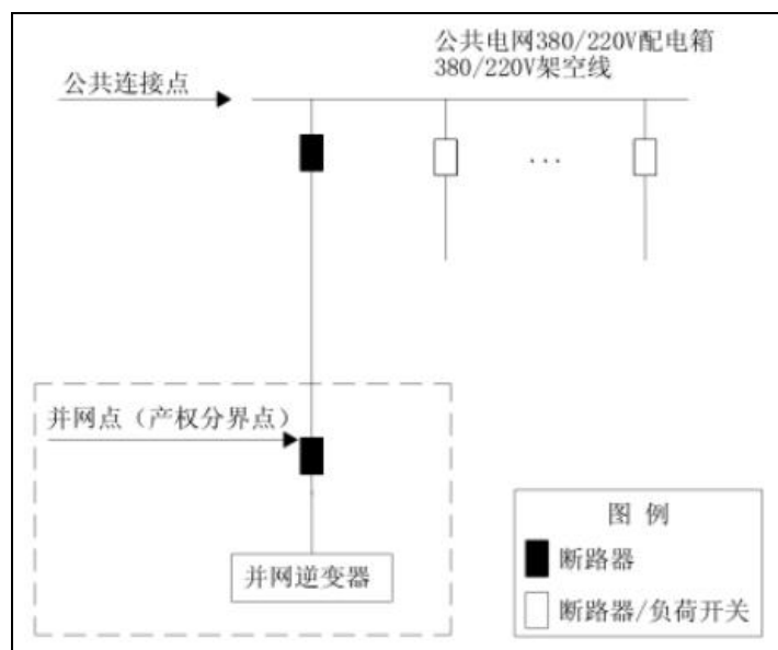
图 3 380V 接入方案三
