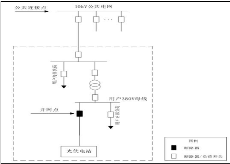
图 1 380V 接入方案一
