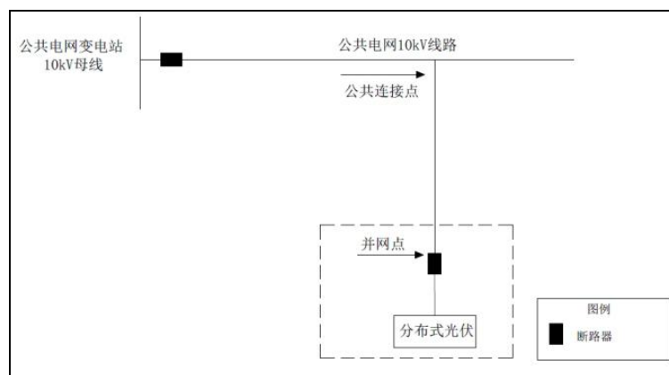
图 4 10kV 接入方案一
